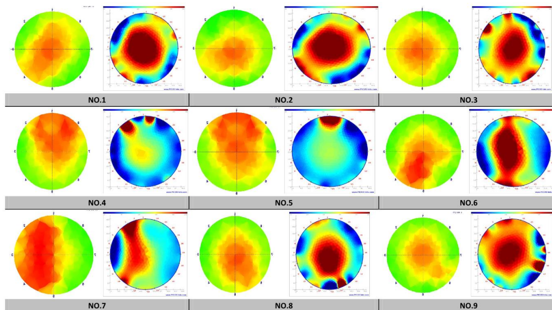
圖 1、SWT 與 ERT 之斷層影像比較
